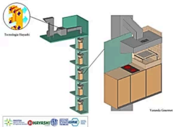
Sistema de Exaustão Varanda Gourmet
